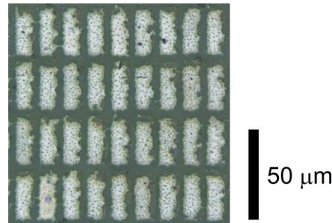
(b) カット金属ワイヤーからなるメタアtomの拡大写真
