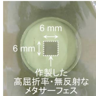
(a) 高屈折率・無反射なメタサーフェスの全体写真
